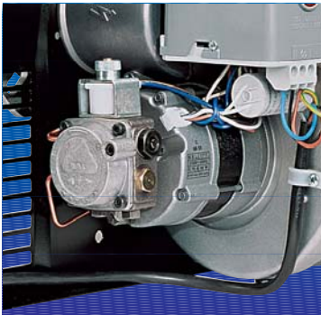
燃料泵
